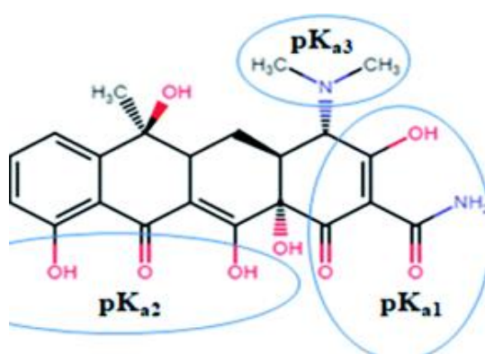
Рис. 1. Будова молекули тетрацикліну (a) і діаграма розподілу протеолітичних форм тетрацикліну в розчині в залежності від pH (b).
