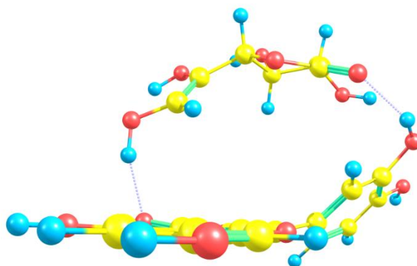
Рис. 3 — Оптимізована структура parallel-комплексу
