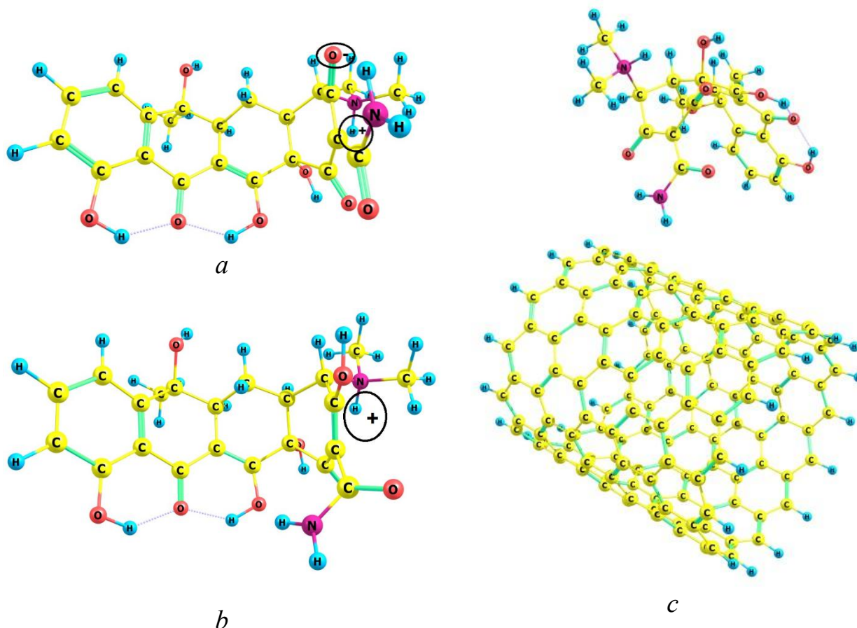
Рис 2. Цвітер-іонна (а) та катіонна (b) форми тетрацикліну. Взаємодія протонованої форми тетрацикліну з фрагментом вуглецевої нанотрубки (с).
