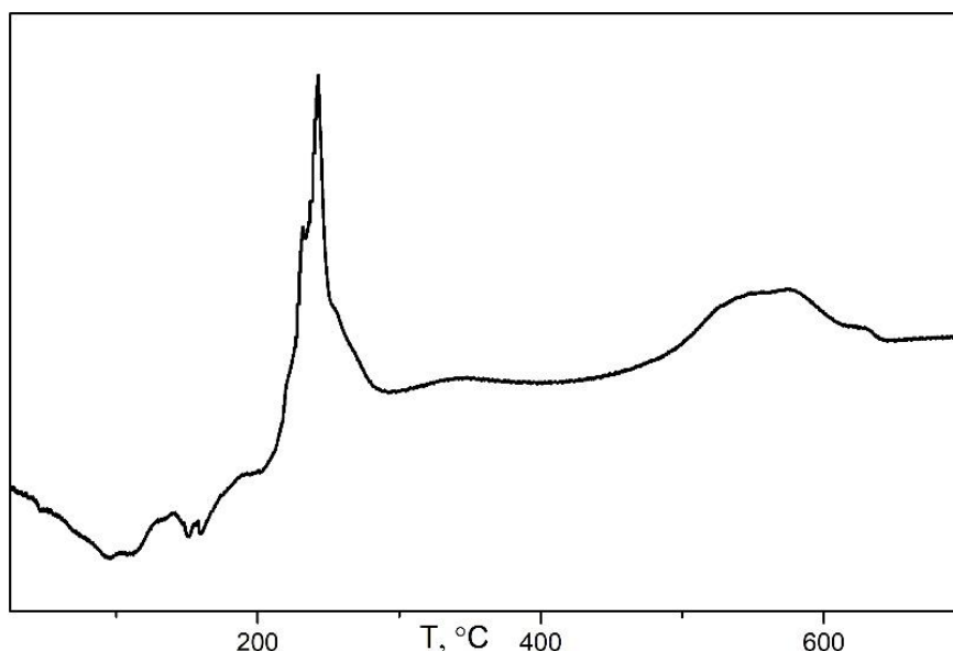
1. ábra. A 100^\circ\text{C} -on szárított \text{LaFeO}_3 gél melegítési görbéje.
