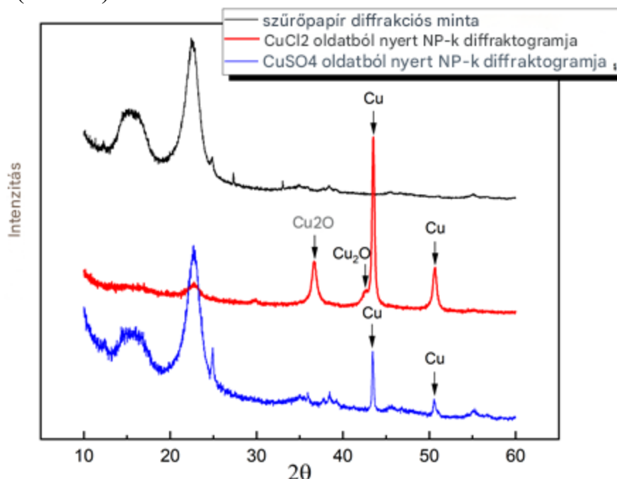
1. ábra. CuSO 4 , CuCl 2 oldatokból nyert NR-k és a szűrőpapír diffraktogramja
