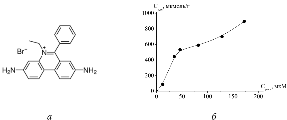
Рисунок – Структурна формула етидій броміду (а) та залежність величини його адсорбції на поверхні ДНК-вмісного діоксиду титану від концентрації сорбату (б). Вміст ДНК на поверхні діоксиду (C ОКС = 1 г/л) титану 0,03 г/л при C ЕТ =20–200 мкМ.
