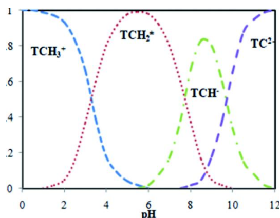
Рис. 1. Будова молекули тетрацикліну (a) і діаграма розподілу протеолітичних форм тетрацикліну в розчині в залежності від pH (b).
