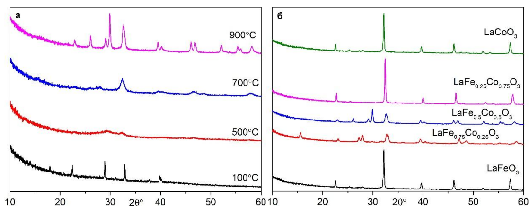
2. ábra. (a) A \text{LaFe}_{0.5}\text{Co}_{0.5}\text{O}_3 összetételű minták diffraktogramjai különböző hőkezelési hőmérsékleteken; (b) a \text{LaFe}_x\text{Co}_{1-x}\text{O}_3 összetételű minták diffraktogramjai 900 °C-on végzett hőkezelést követően.
